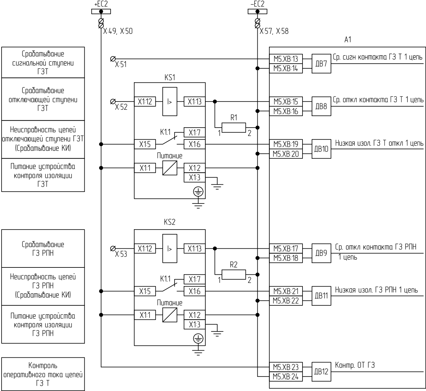
Цепи оперативного тока ГЗ Т
